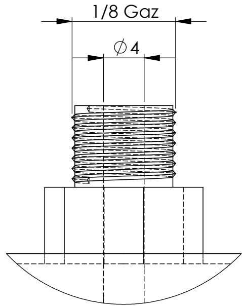
DÉTAIL A ECHELLE 8 : 3
